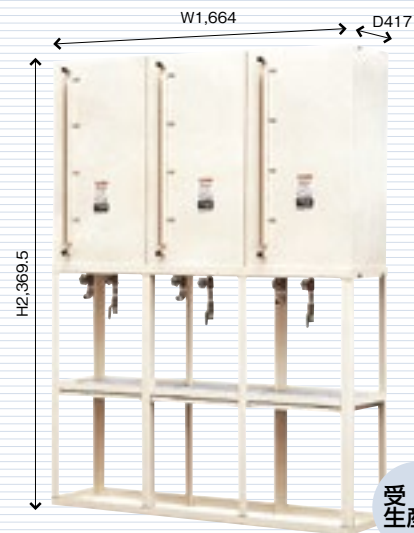
□3連式ウォールタンク(3/4ボールバルブ付) 容積：248ℓ×3 容量：230ℓ×3 重量：276.9kg
