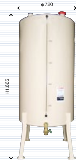
□500丸型(1インチバルブ付) 容積：523ℓ 容量：490ℓ 重量：71kg
