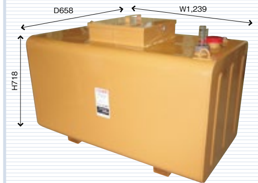
□廃油専用500角型
